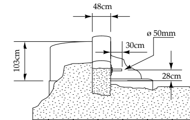
VIEW A-A
