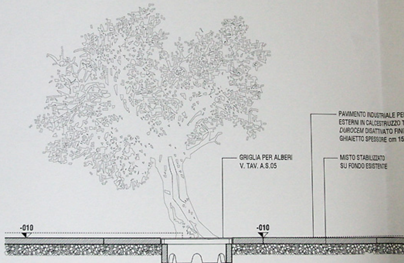
SEZIONE C-C: STATO DI PROGETTO RAPP. 1: 50
