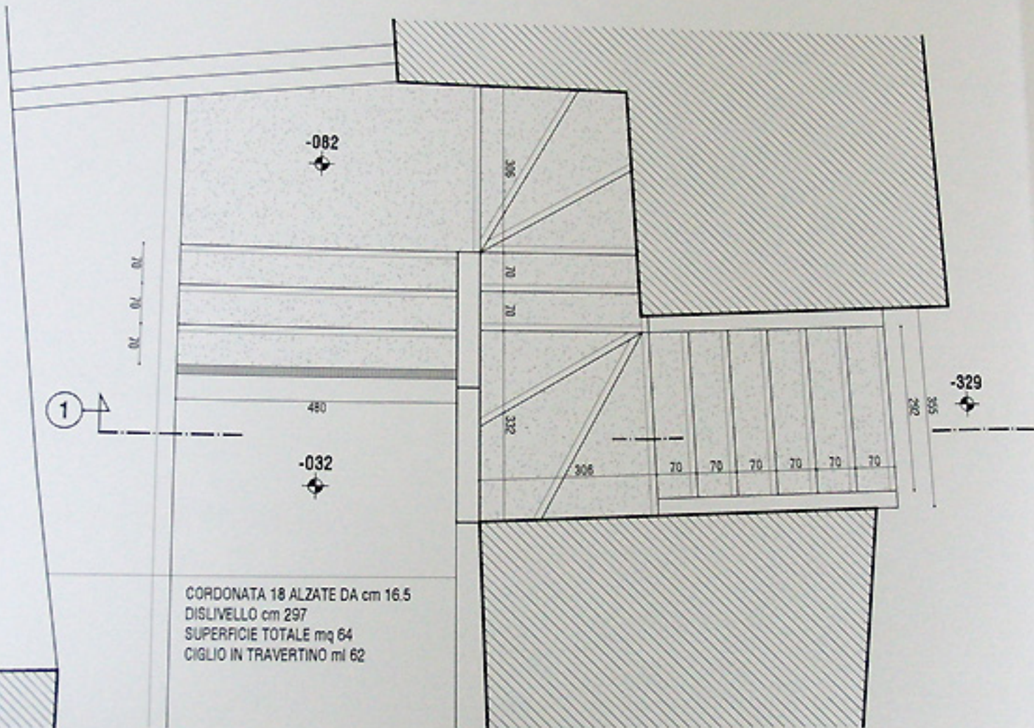
CORDONATA: PIANTA RAPP. 1: 100
